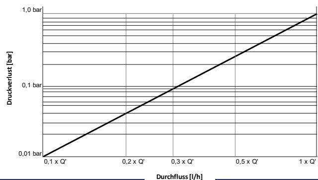
Typische Druckverlustkurve
