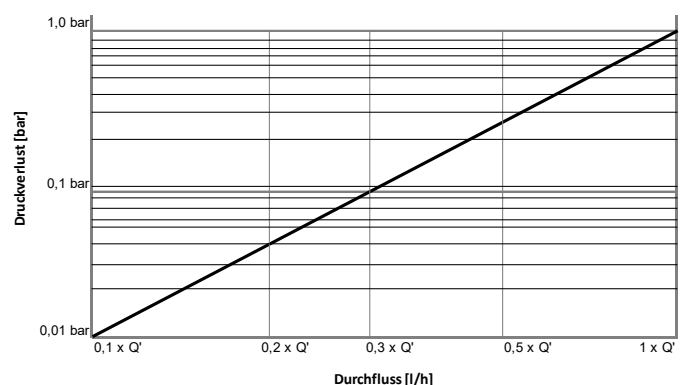
Typische Druckverlustkurve
