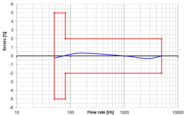
Typische Fehlerkurve für Q 3 4 R80H
