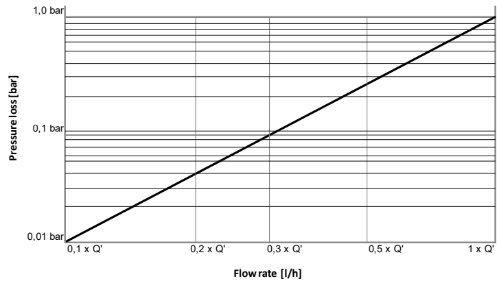
Typische Druckverlustkurve
