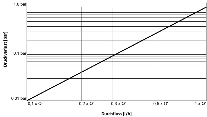
Typische Druckverlustkurve
