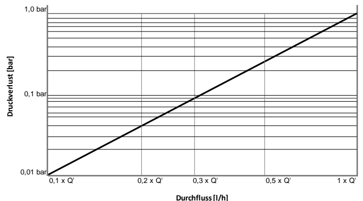
Typische Druckverlustkurve
